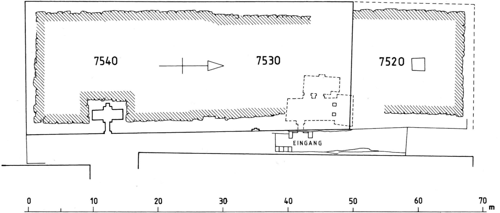
Abb. 3. Die Anlagen G 7520, G 7530–7540 und G 7530 sub (nach D. Dunham–W. K. Simpson, Mersyankh III, Plan B und C)
